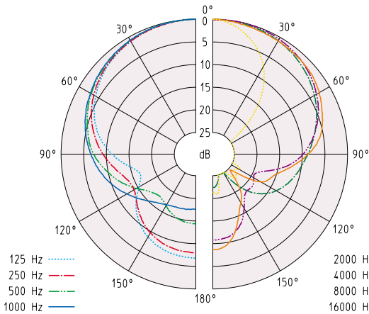
Richtdiagram
