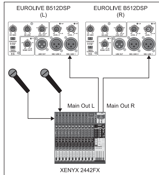
Abb. 4.2: Anschluss eines Mischpults
