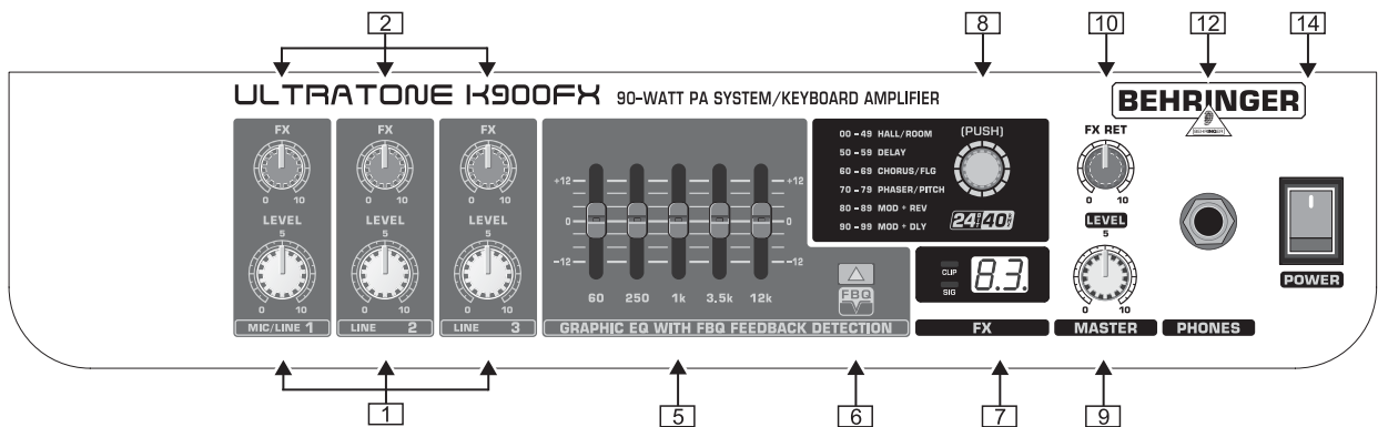
Abb. 2.3: Bedienungselemente auf der Vorderseite (für K900FX und K450FX)
