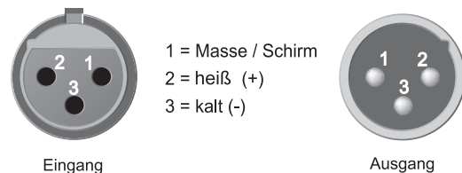
Abb. 4.3: Verkabelung eines XLR-Anschlusses
