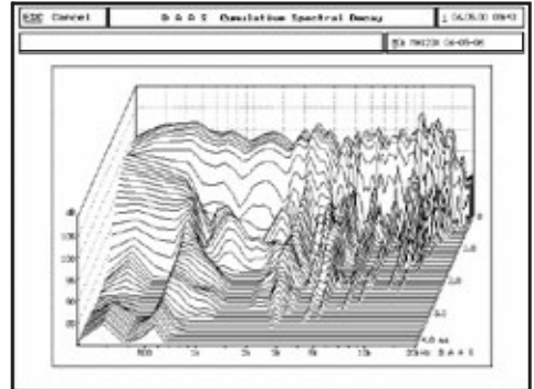
Wasserfall Spektralanalyse
