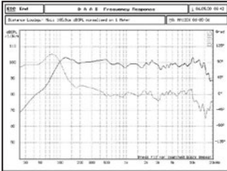
Frequenzverlauf, SPL/2.83v
